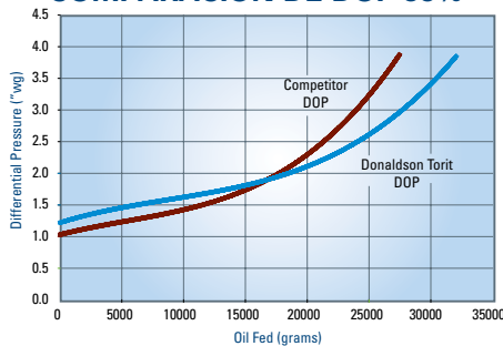
COMPARACIÓN DE DOP 95%**
