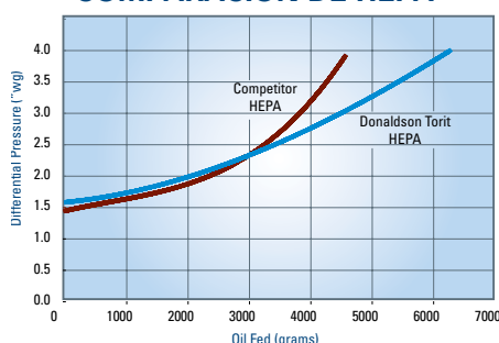
COMPARACIÓN DE HEPA*
